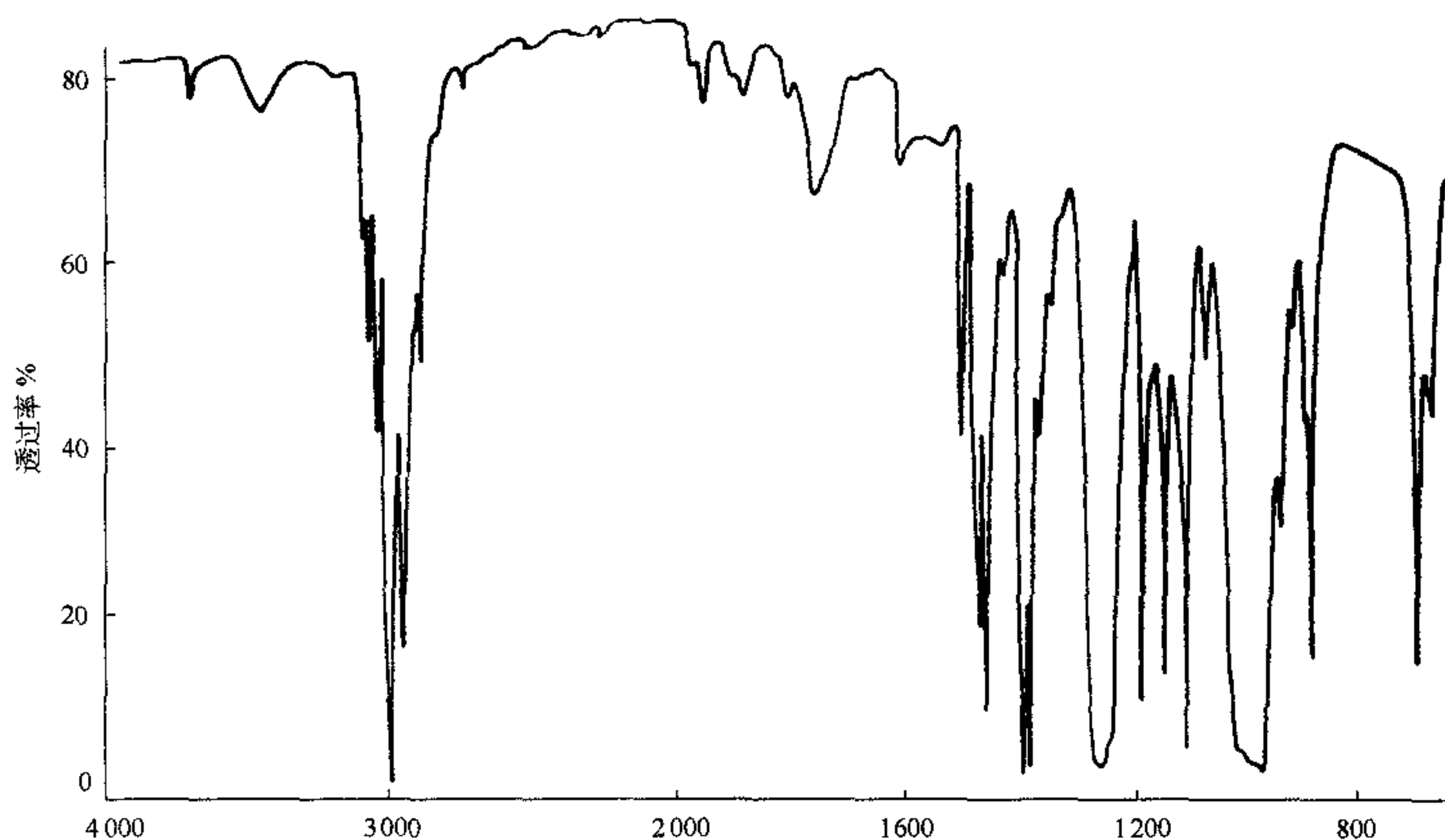
图 1 异稻瘟净的红外光谱图
